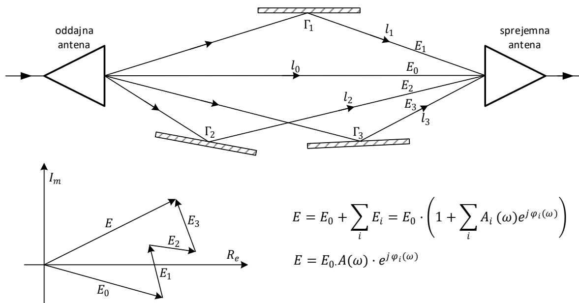
Slika 1: Popačenje prenosne funkcije pri razširjanju radijskih valov po več različnih poteh.
