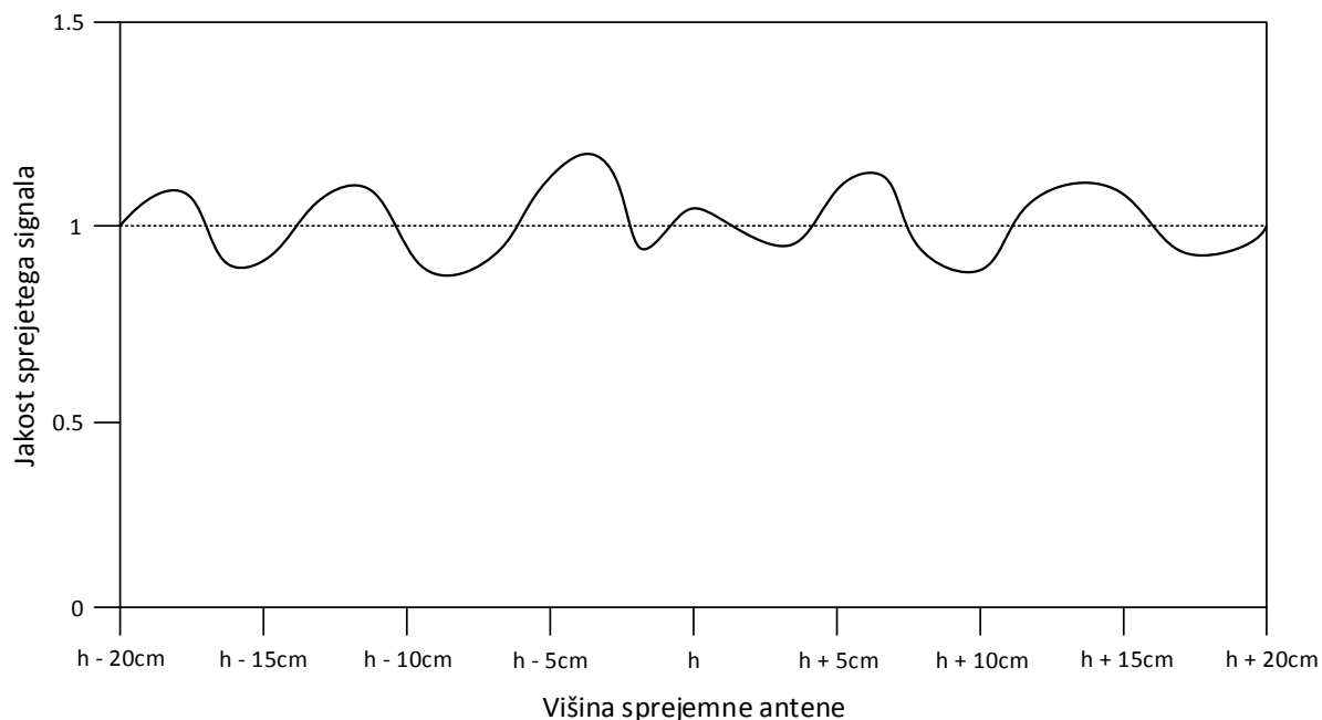
Slika 4: Vpliv odbitih valov na jakost sprejetega signala
