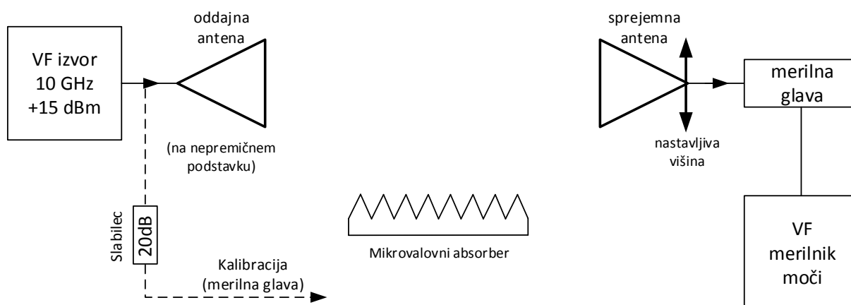
Slika 2: Skica vezave merilnih pripomočkov
