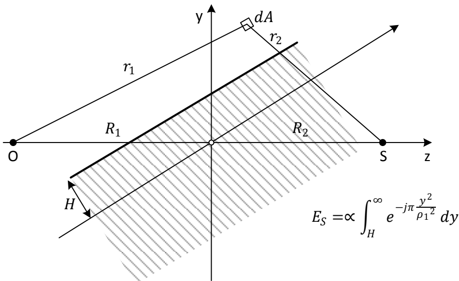
Slika 1: Uklon valovanja na prečni klinasti oviri
