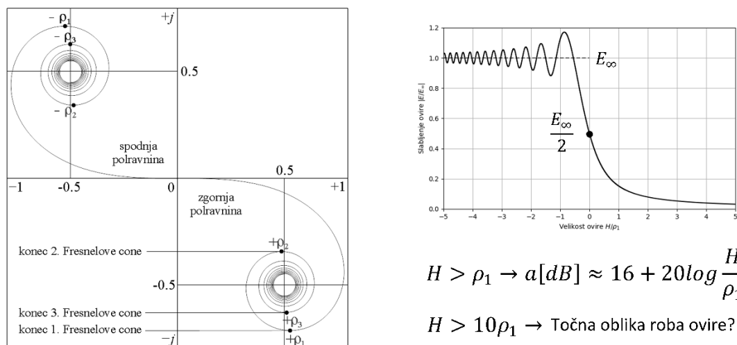
Slika 3: Določanje uklonskega slabljenja klinaste ovire
