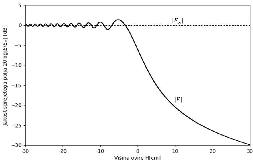
Slika 6: Primer uklonskega slabljenja klinaste ovire
