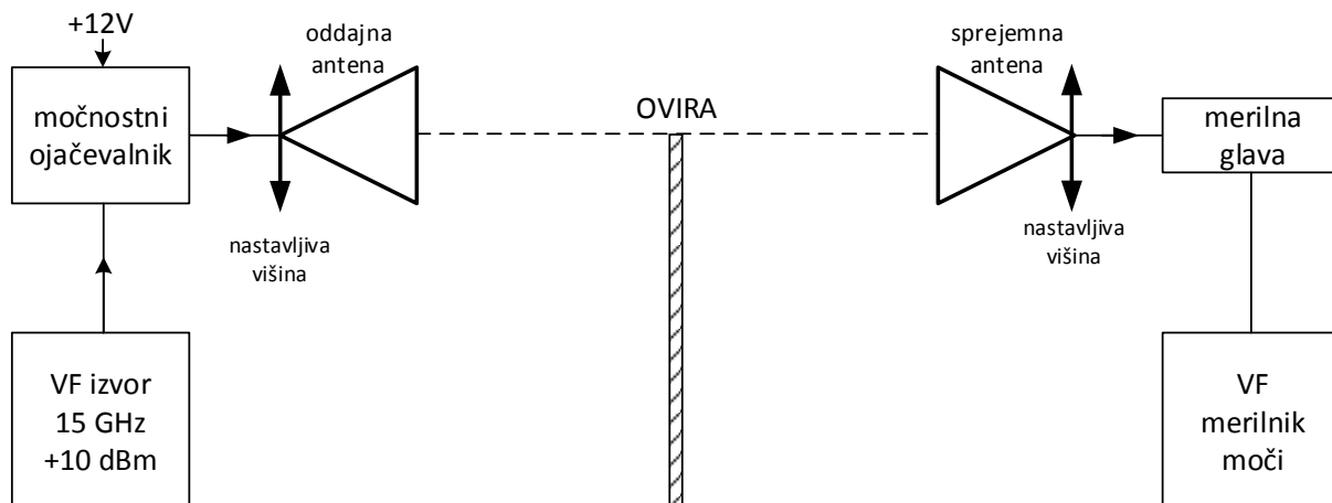
Slika 4: Skica vezave merilnih pripomočkov
