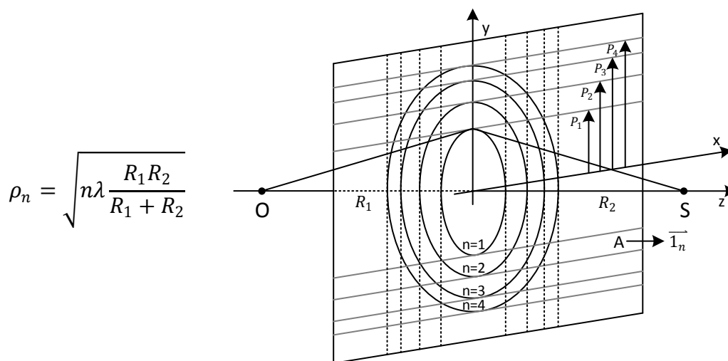
Slika 2: Fresnelovi pasovi
