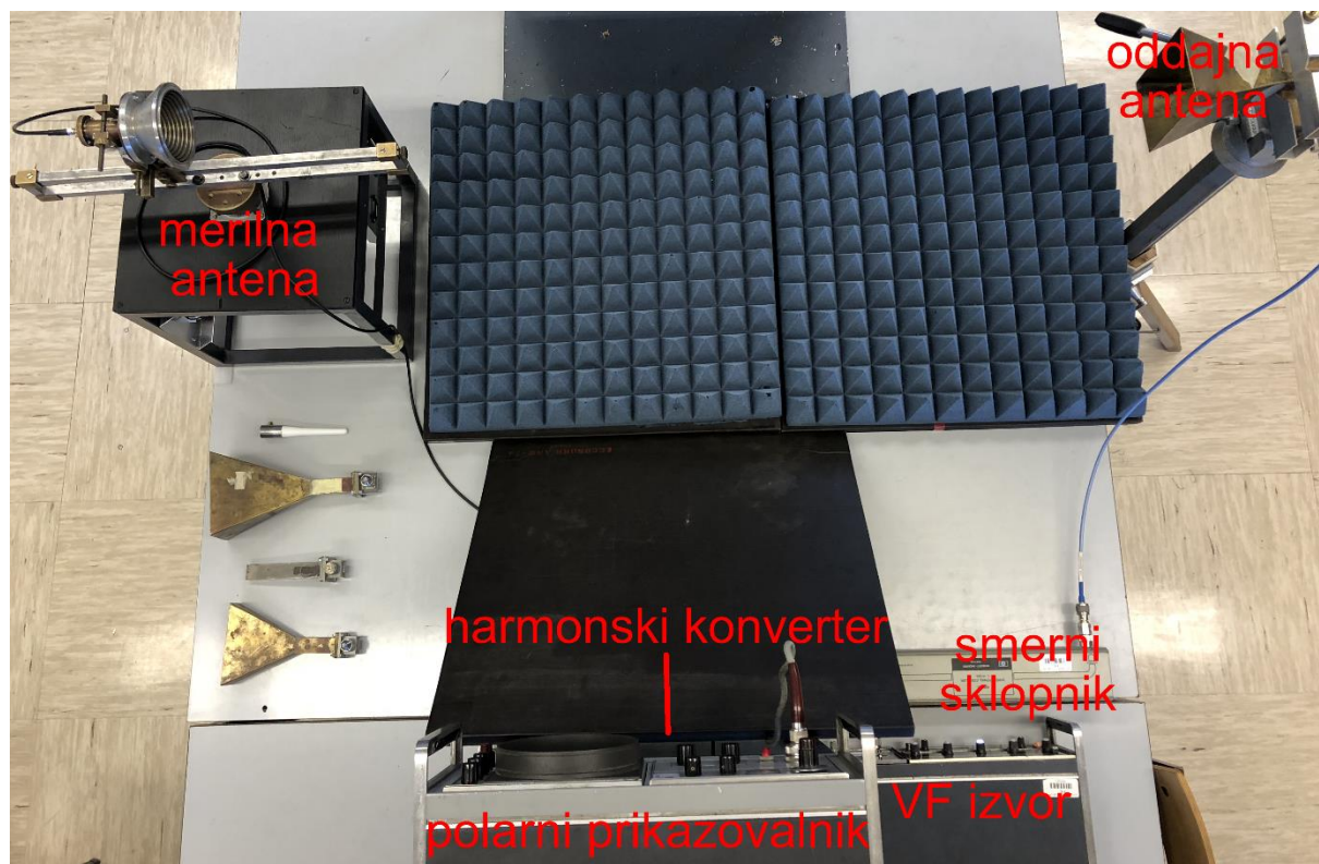
Slika 4: Slika vezave merilnih pripomočkov
