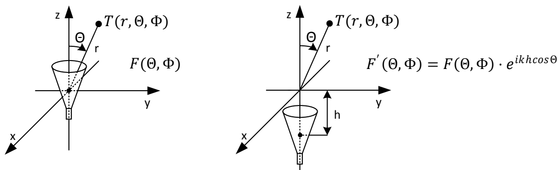
Slika 2: Učinek premika antene po osi z na fazo smerne diagrama
