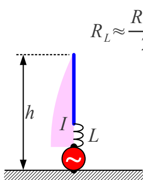
Koncentrirana tuljava
