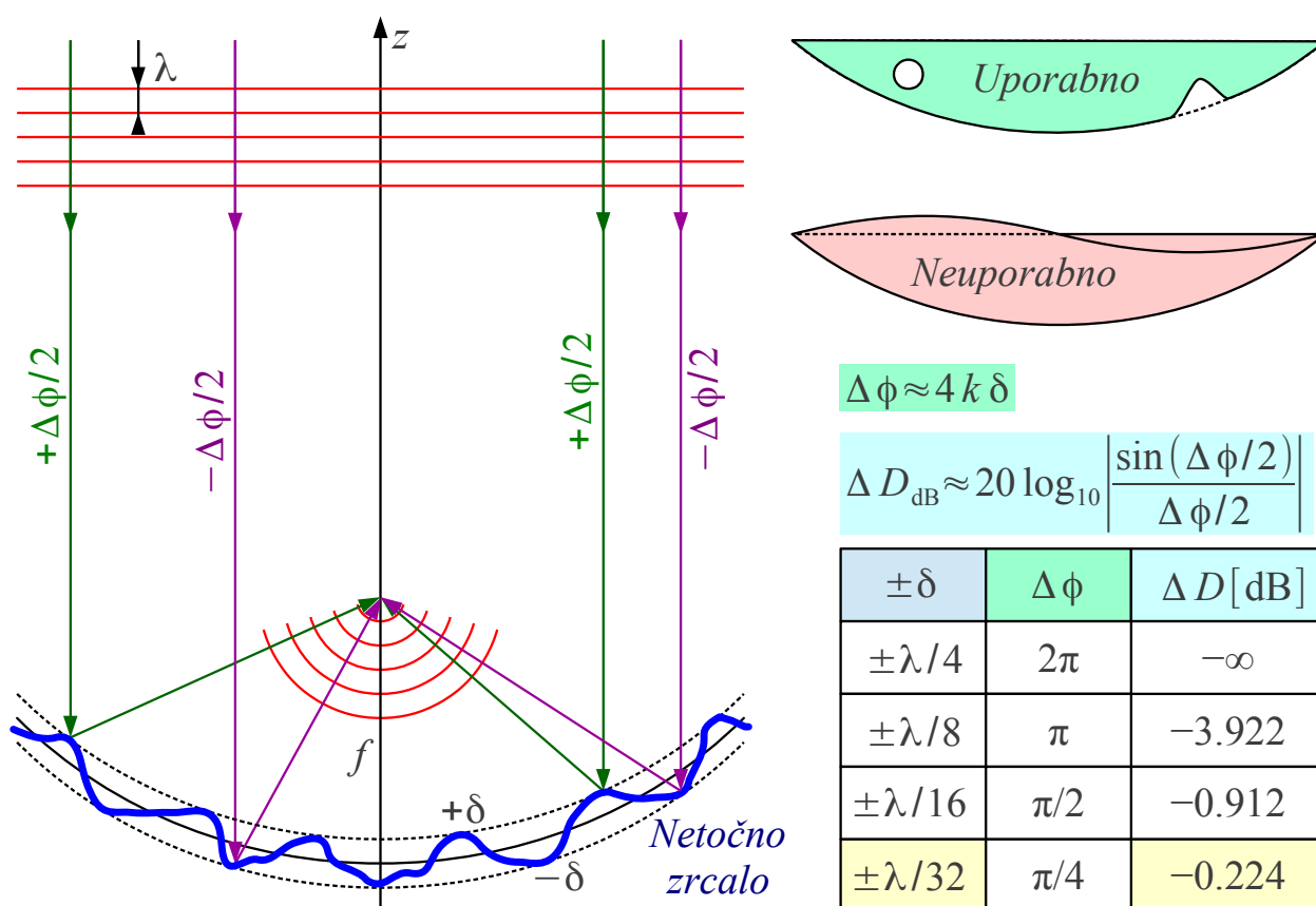
Napake oblike zrcala
