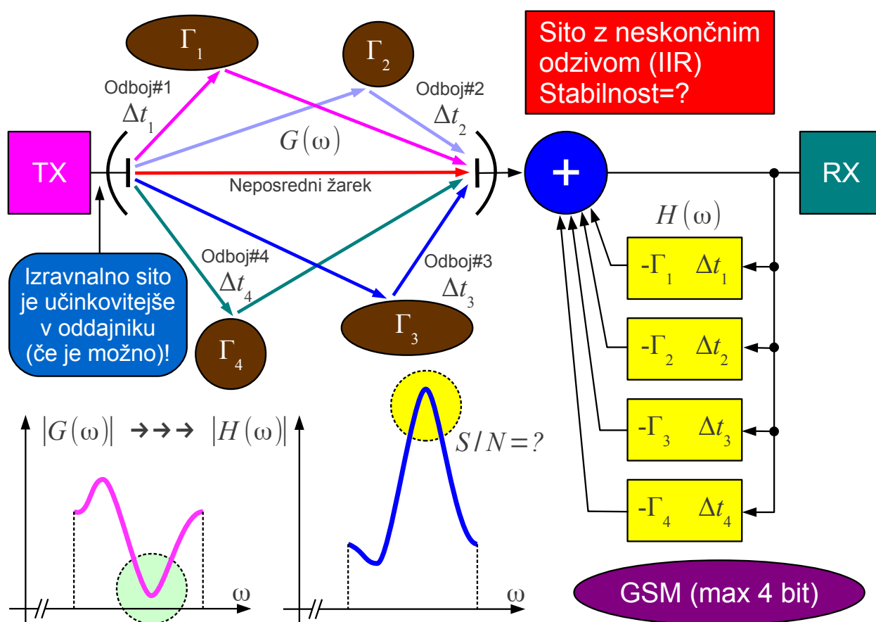
Odpravljanje popačenja večpotja z izravnalnim sitom
