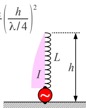
Porazdeljena tuljava
