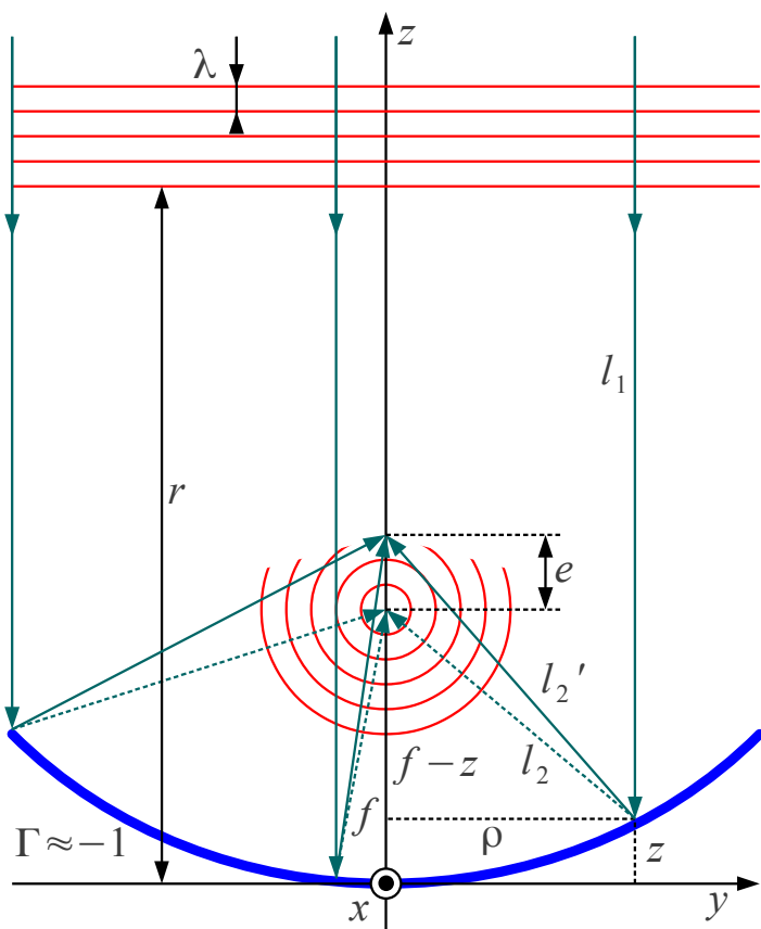
Osni odkik žarilca
