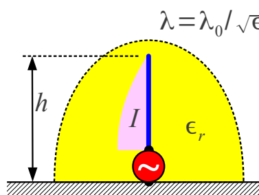
Monopol v dielektriku
