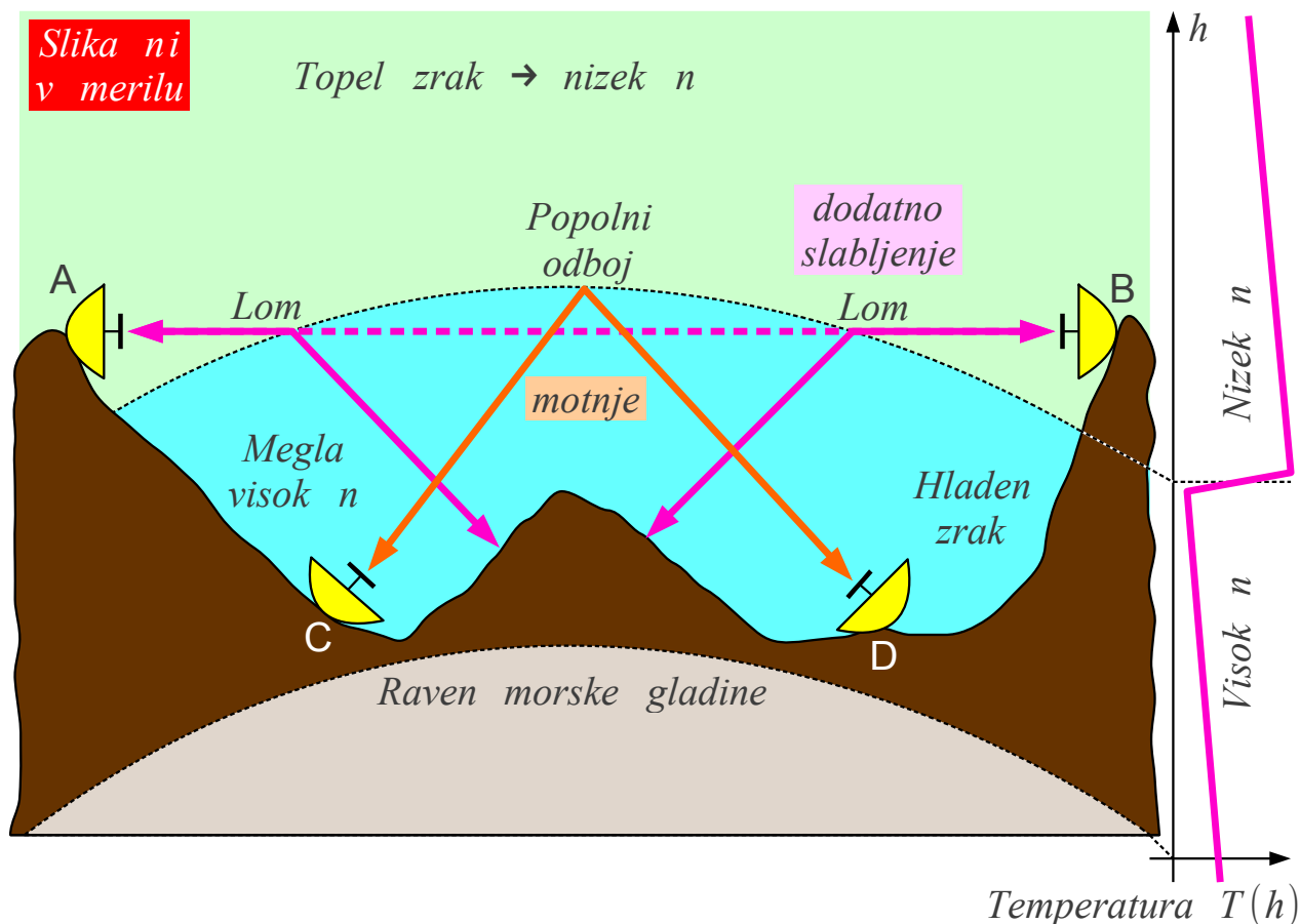
Temperaturna inverzija
