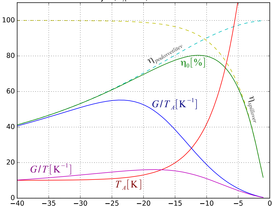
Razmerji G/T_A in G/T zrcalne antene
