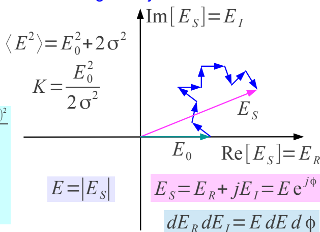
Večpotje z neposrednim žarkom: Rice ( E_0, \sigma ) en velik in mnogo naključnih malih kazalcev
