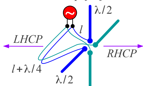
Križna dipola kvadraturno napajanje
