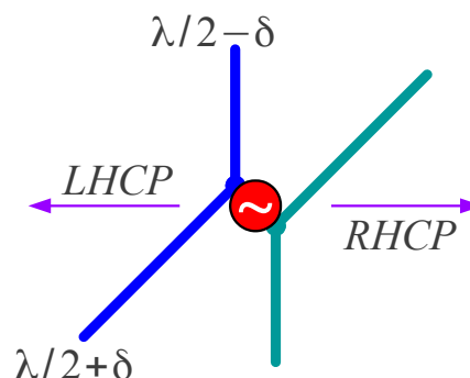
Križna dipola različnih dolžin
