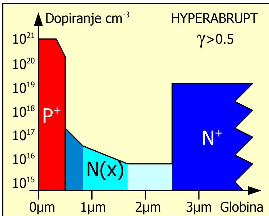
Kapacitivnost varikap diode v odvisnosti od profila dopiranja
