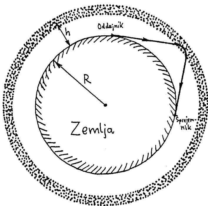
Slika 5 - Najvišja frekvenca popolnega odboja (MUF).
