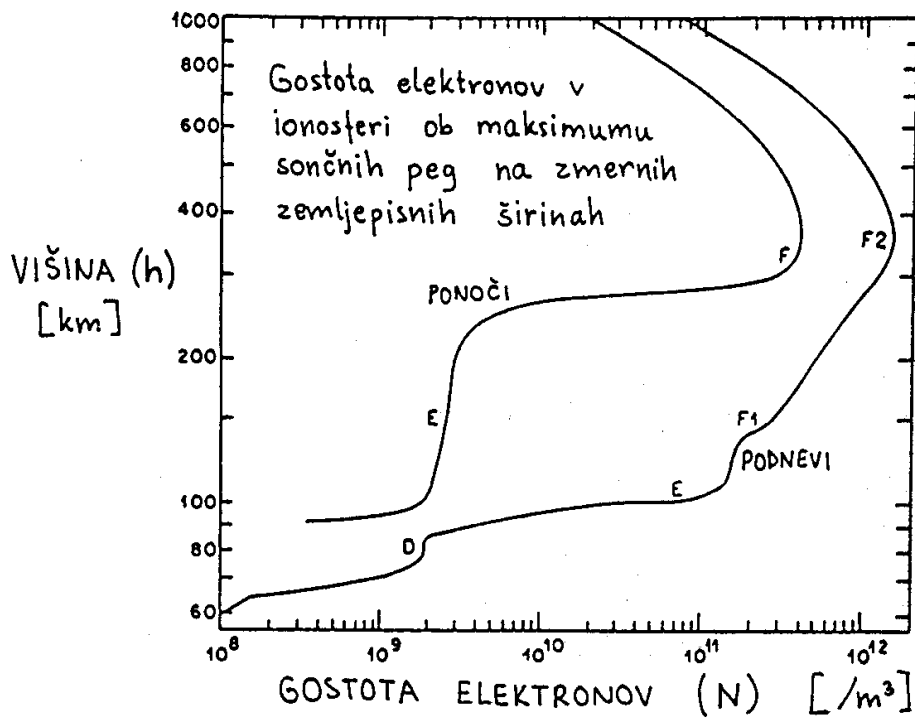
Slika 1 - Plasti zemeljske ionosfere.
