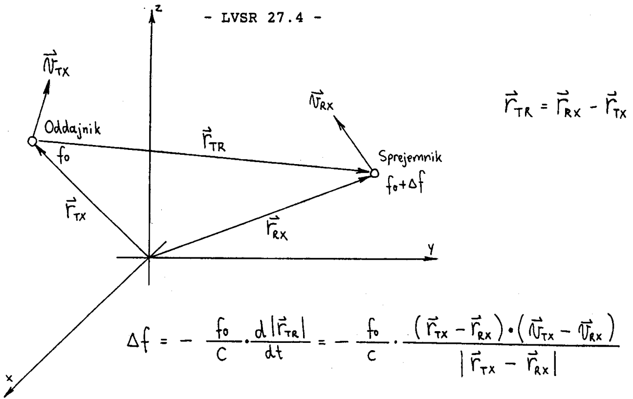
Slika 1 - Doppler-jev pomik frekvence sprejetega signala.
