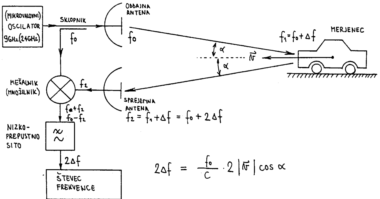
Slika 2 - Običajna izvedba Doppler-jevega radarja.
