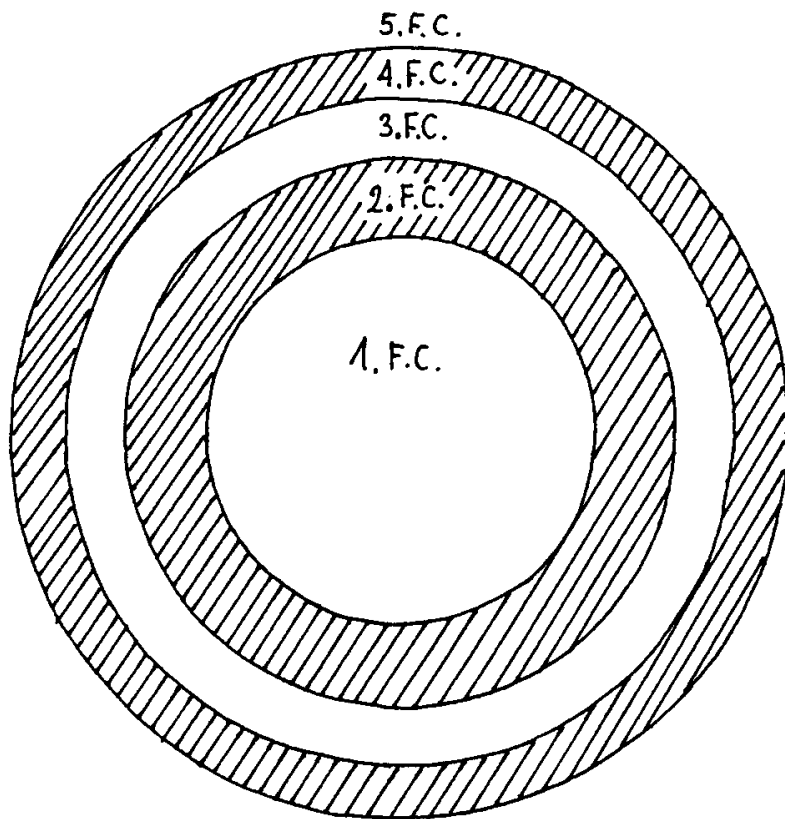
Slika 4. - Difraktor s senčenjem okroglih Fresnelovih con.
