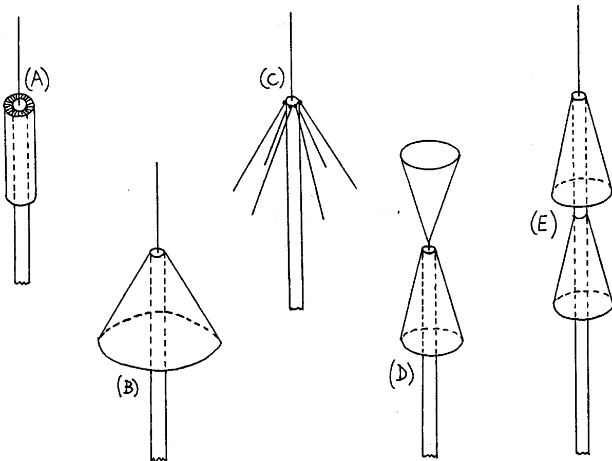
Slika 1 - Tokovi na pokončni anteni.
