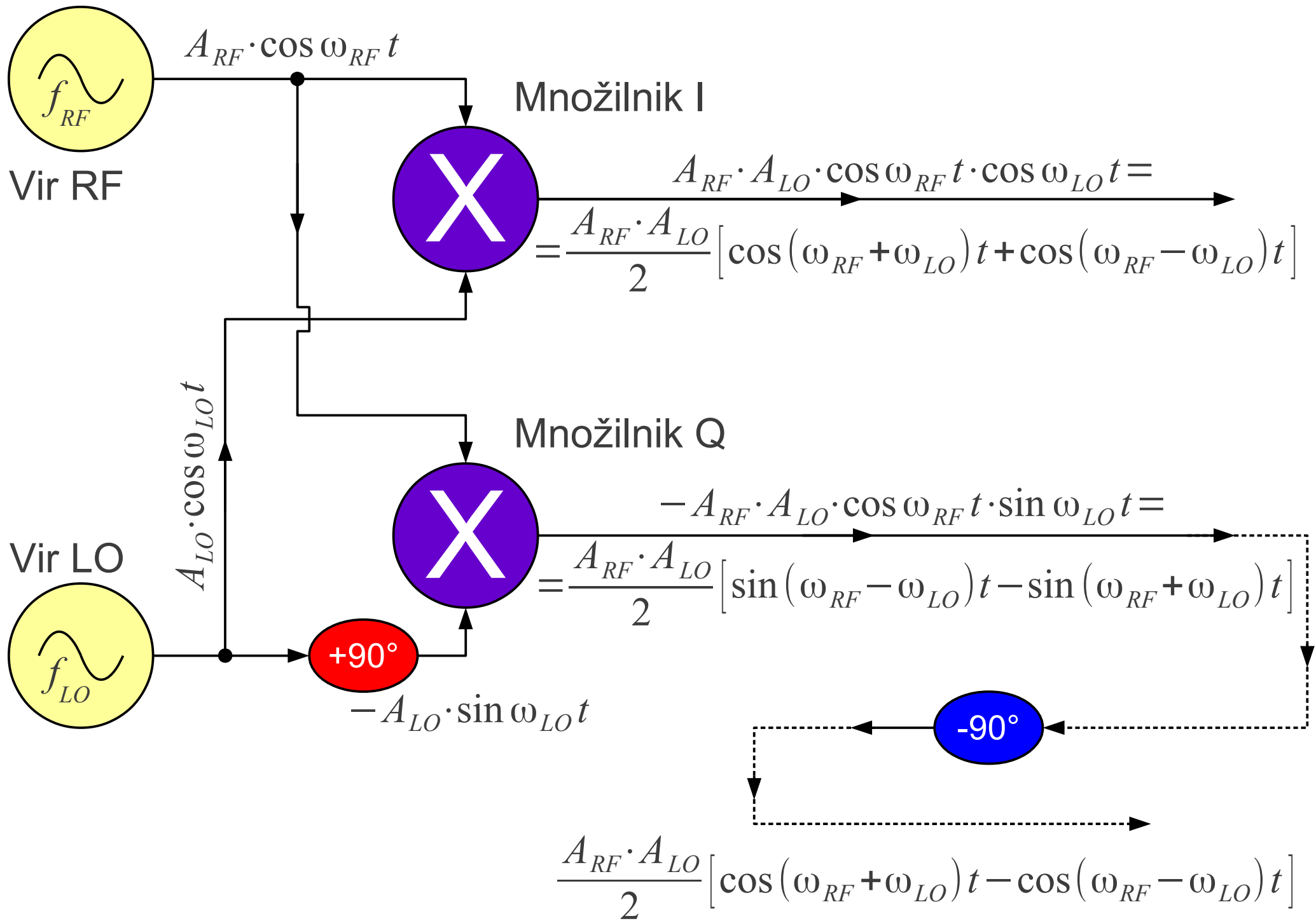
Kvadrturni mešalnik
