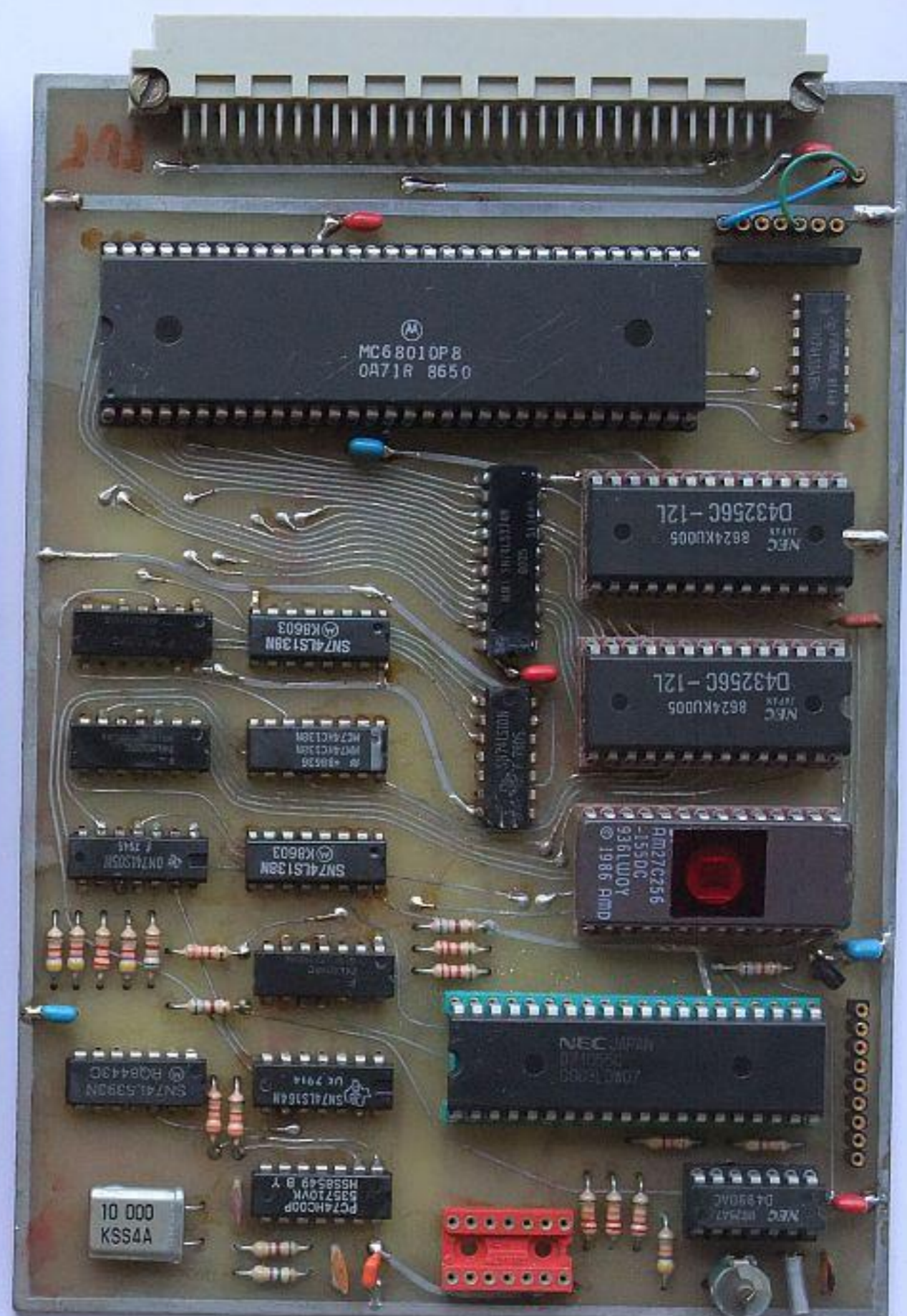
Računalnik z MC68010 (1986)
