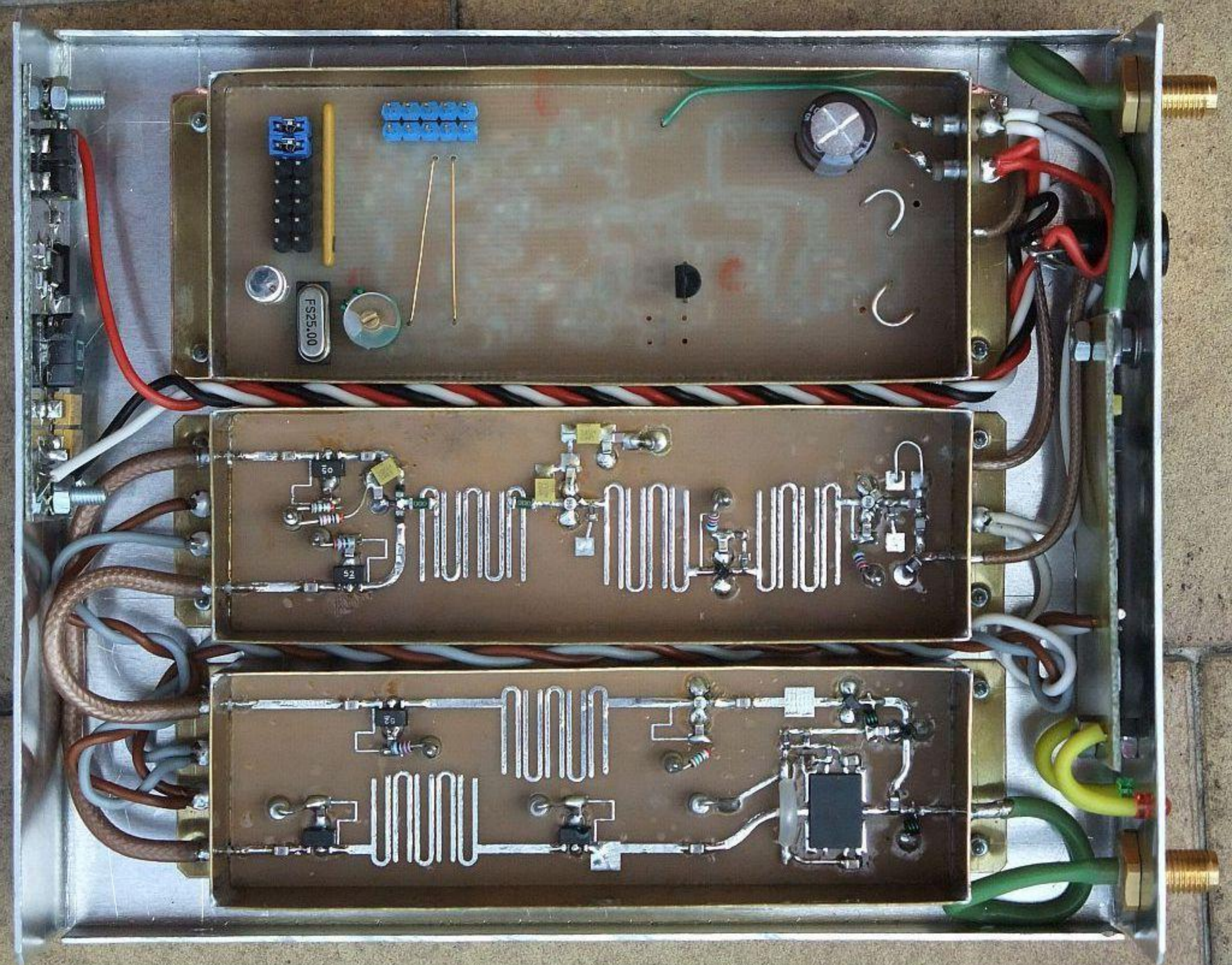
Radijska glava 3.4GHz 2W 100km @10Mbps (2014)
