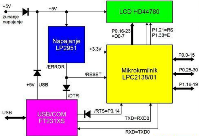
Vezava mikrokrmilnika LPC2138/01
