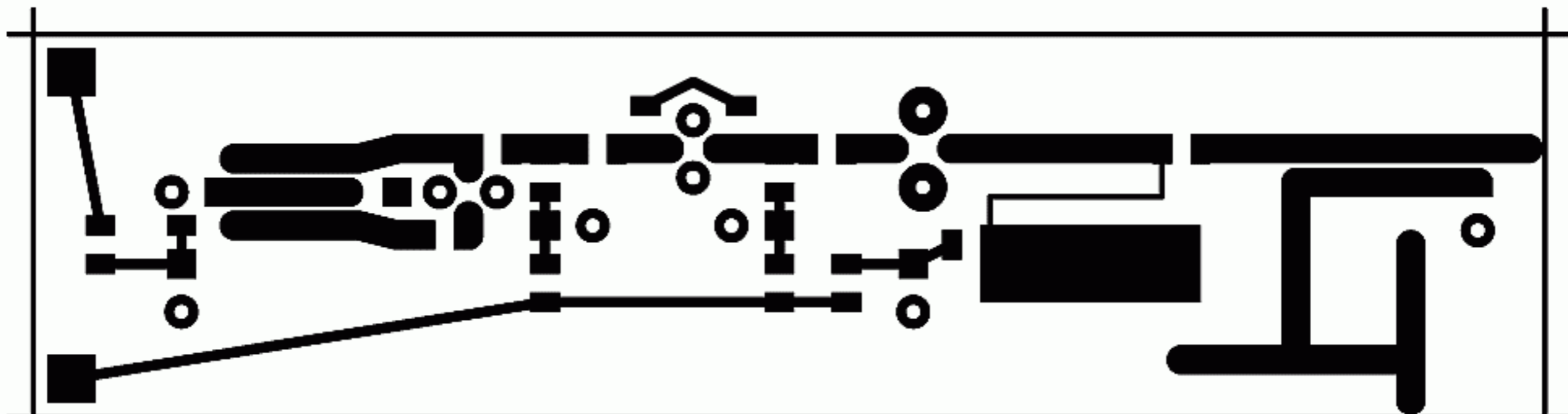
VCO 4.3GHz teflon 19mils \epsilon_r=2.43 80x20
