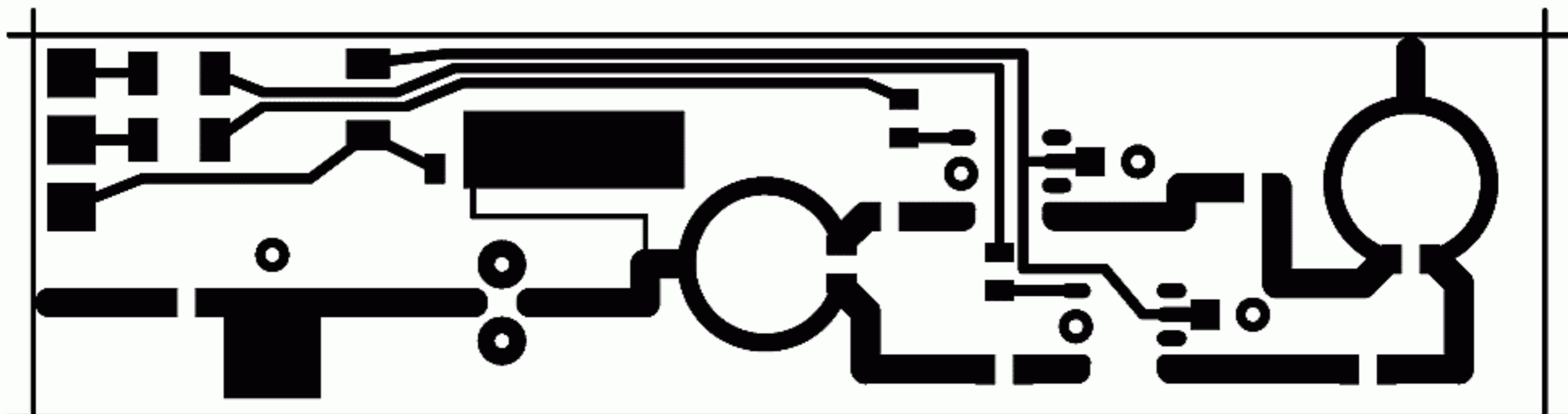
IQmix 4.3GHz teflon 19mils \epsilon_r=2.43 80x20
