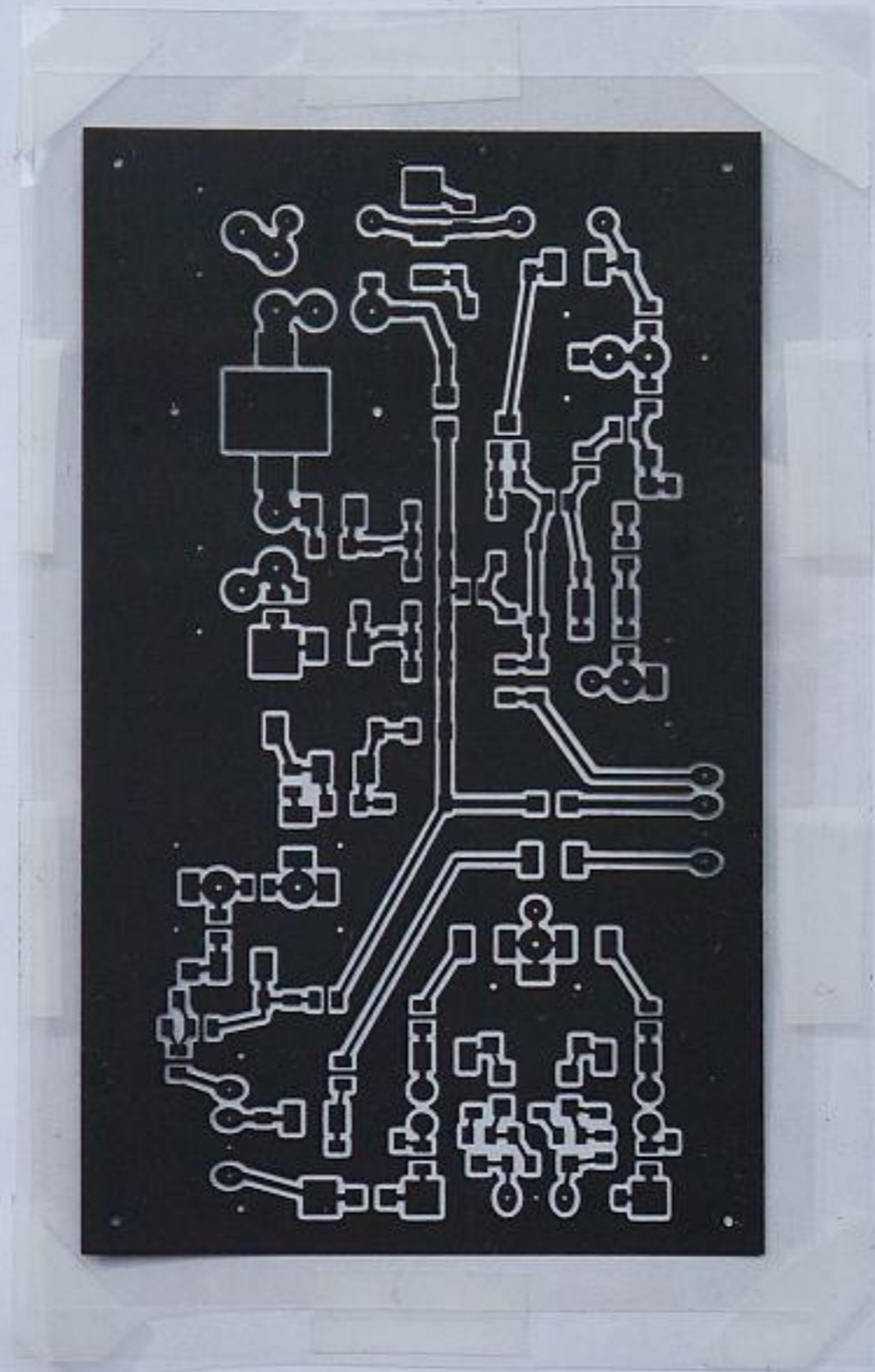
Film za fotopostopek (dvojno tiskanje)
