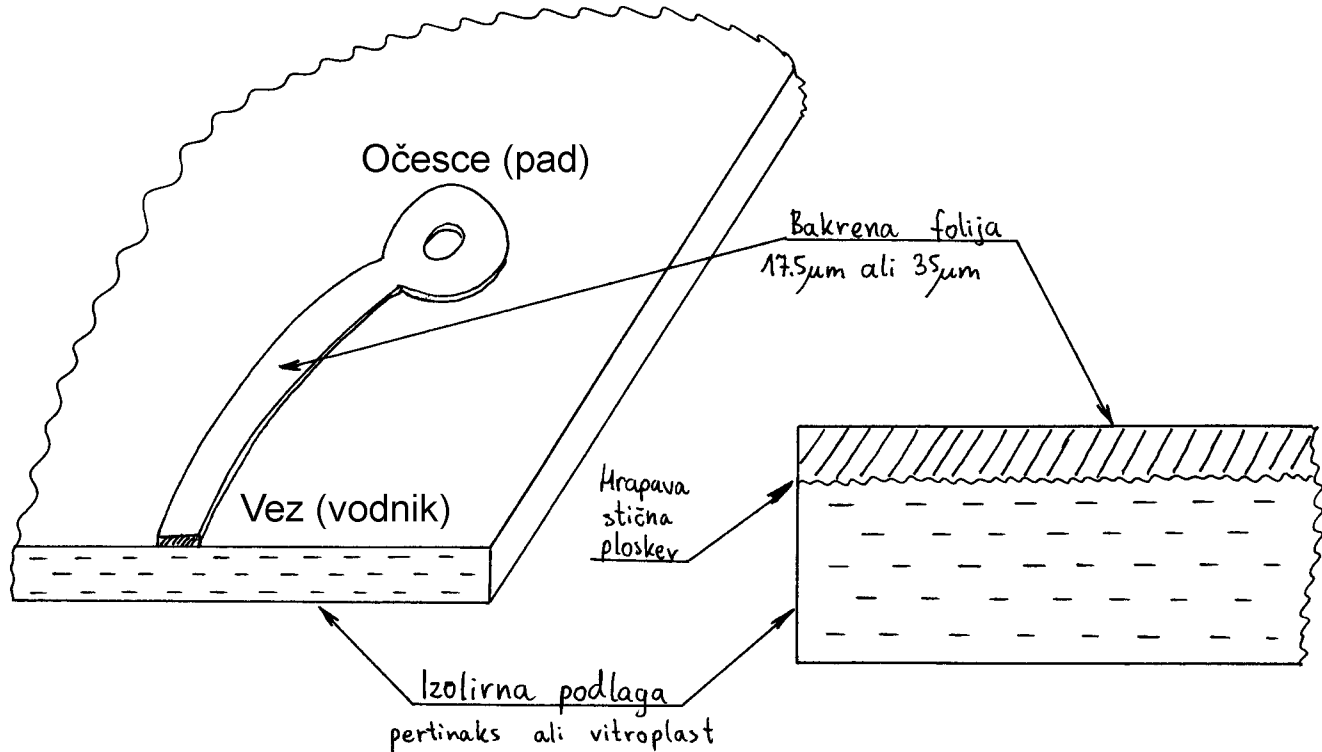
Prerez laminata za enostransko tiskano vezje
