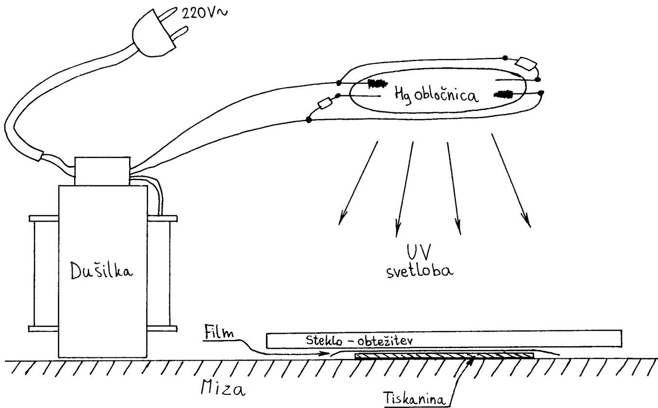
Namestitev filma in laminata pod UV svetilko
