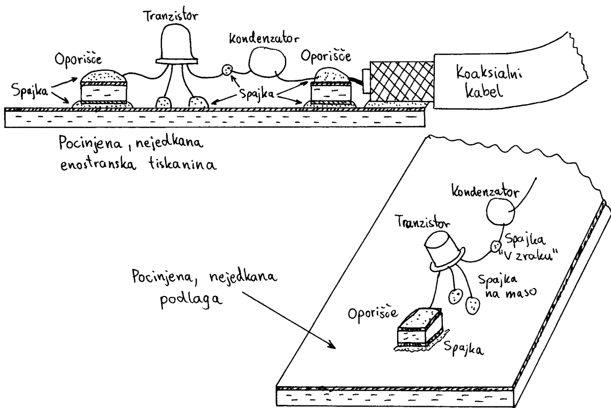
Prototip na nejedkani tiskanini z oporišči
